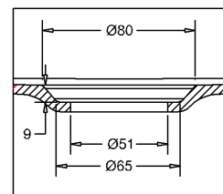
C SCALE 1:2
