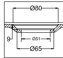
C SCALE 1:2
