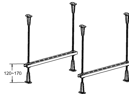
C SCALE 1:2
