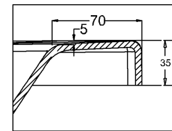
D SCALE 1:2
