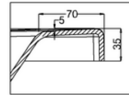
D SCALE 1:2
