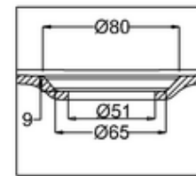
C SCALE 1:2
