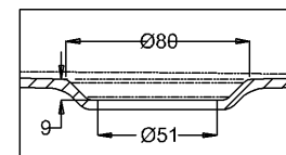
C SCALE 1:2
