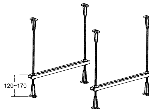
D SCALE 1:2
