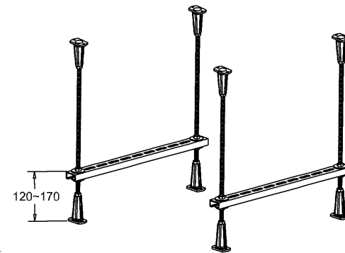
D SCALE 1:2
