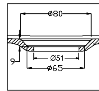
C SCALE 1:2
