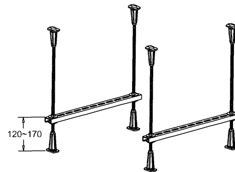
C SCALE 1:2
