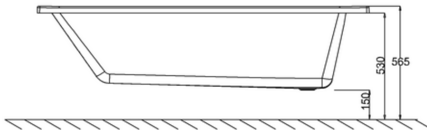
A-A
