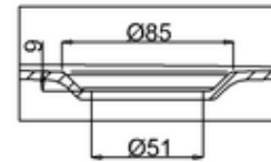
C SCALE 1:2
