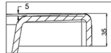
D SCALE 1:2
