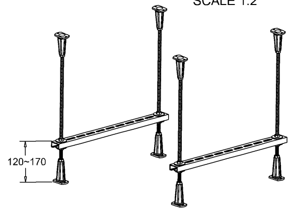
C SCALE 1:2
