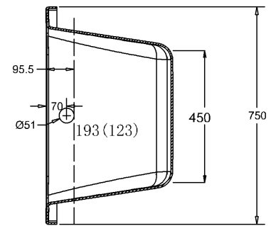
B-B
