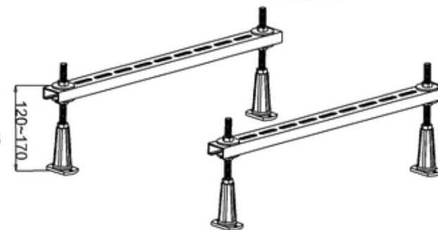
D SCALE 1:2
