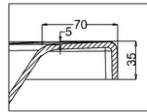
D SCALE 1:2
