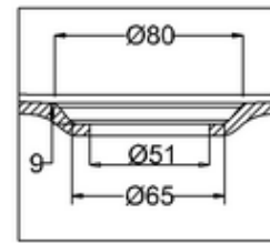
C SCALE 1:2
