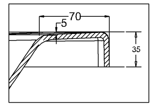
D SCALE 1:2
