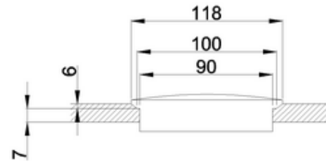
B-----B
