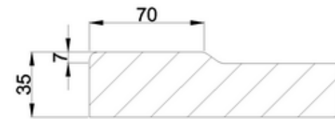
A-----A
