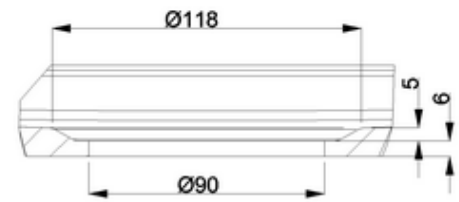
C SCALE 0,5
